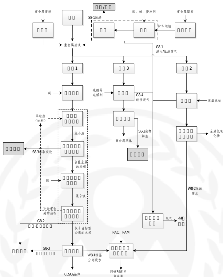
图 5 重金属废物处置工艺流程图
