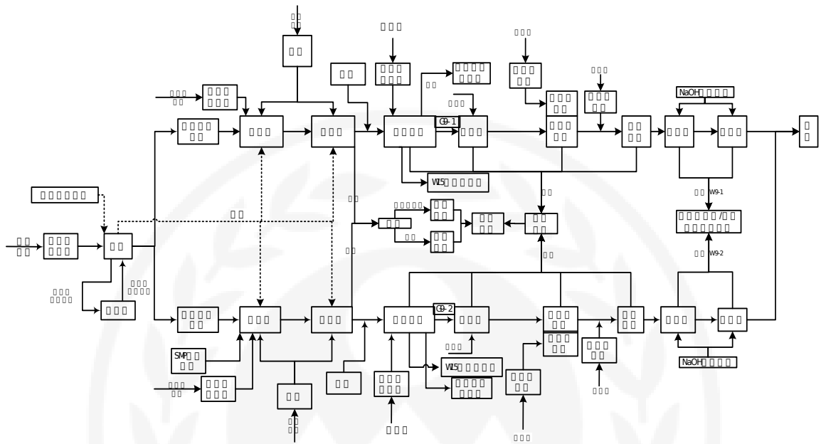
图 1 焚烧处置工艺流程图
