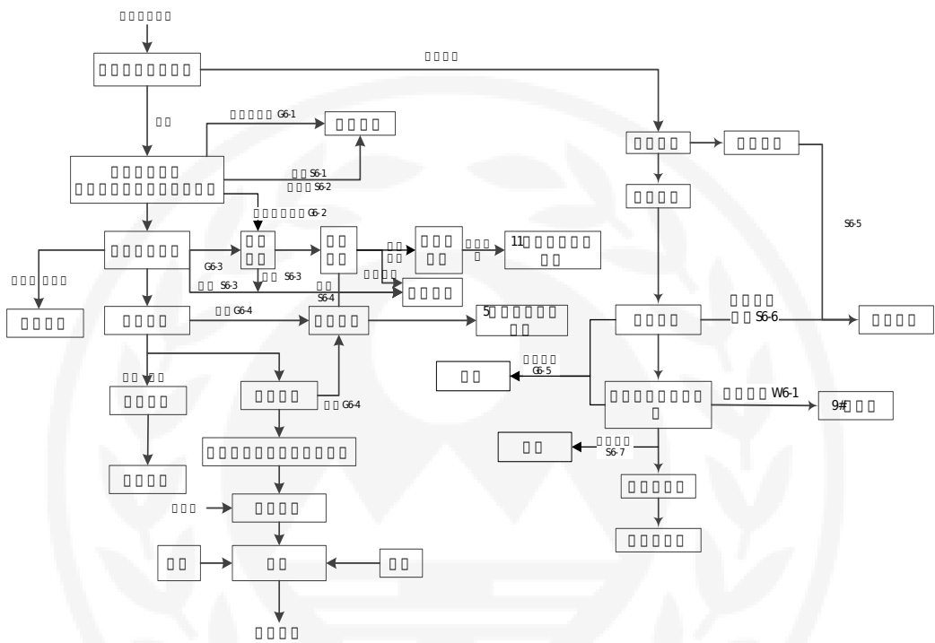
图 8 废包装容器处置工艺流程图
