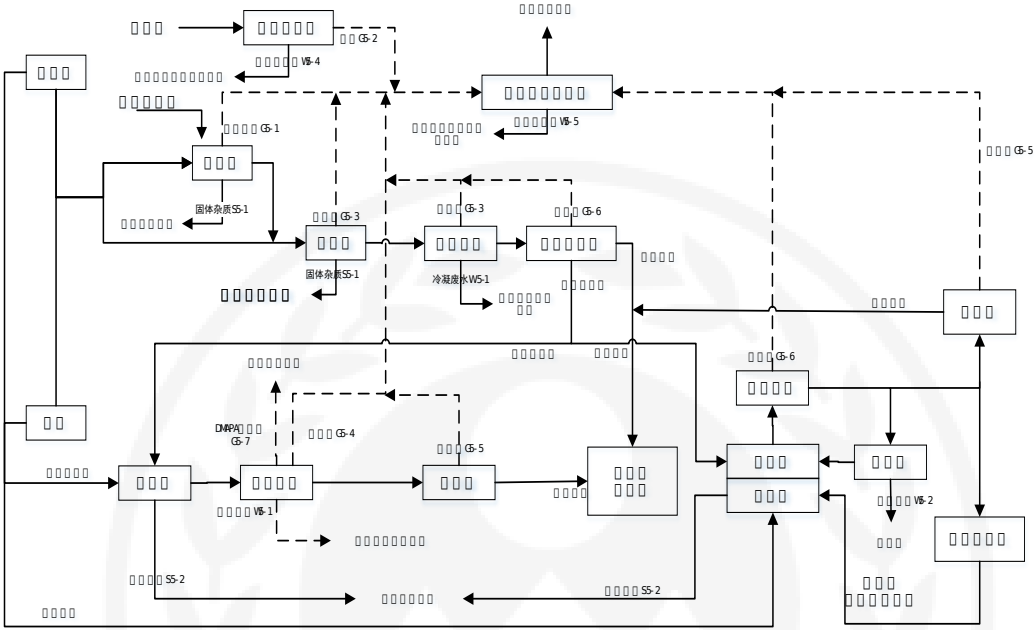
图 4 废有机溶剂处置工艺流程图
