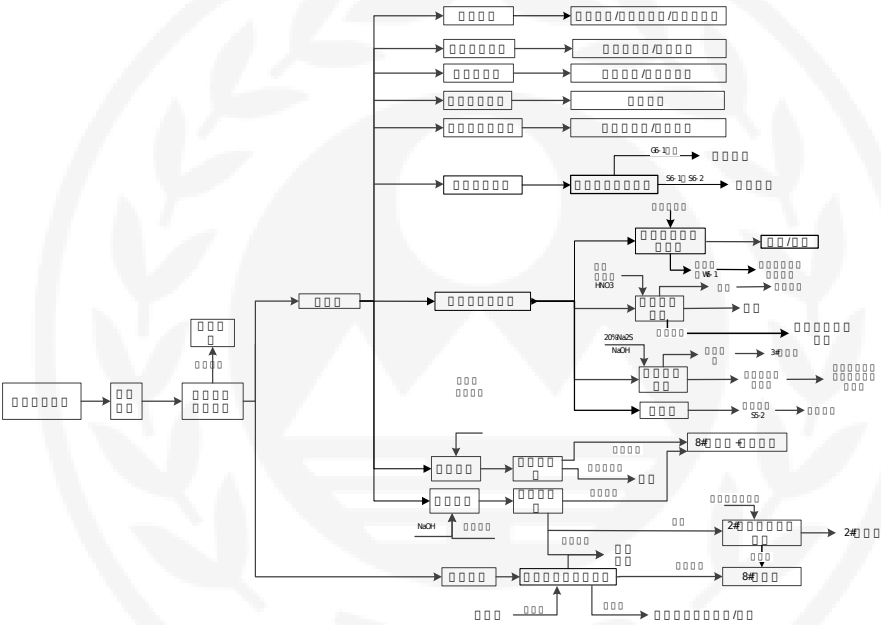
图 7 综合废物处置工艺流程图
