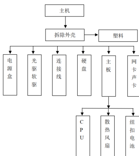
废主机拆解工艺流程
