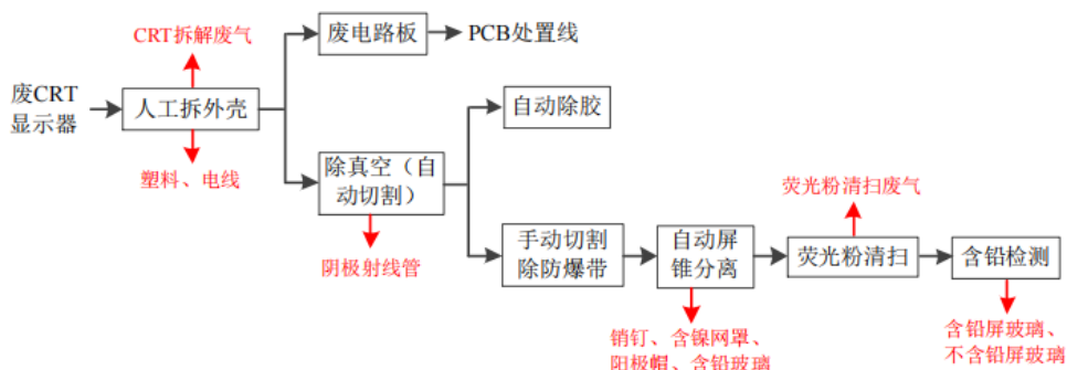
废电视、电脑、CRT 显示器处置流水线
