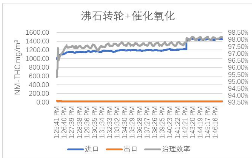
图 6.3-1 企业 A 进出口浓度及处理效率
