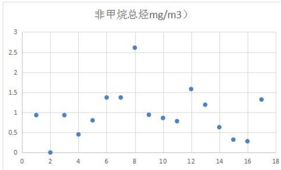
图 6.4-2 厂区非甲烷总烃达标情况
