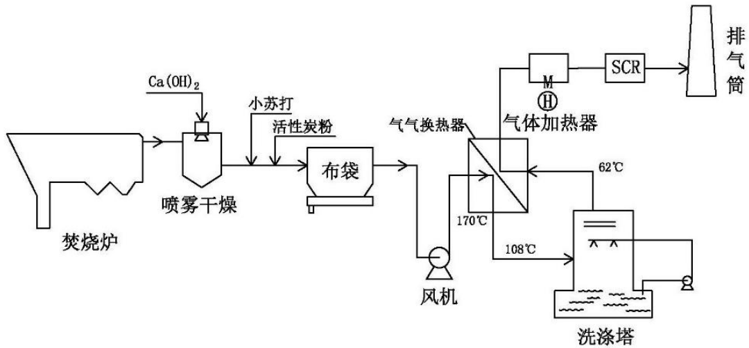
图5 D型生活垃圾焚烧烟气净化系统
