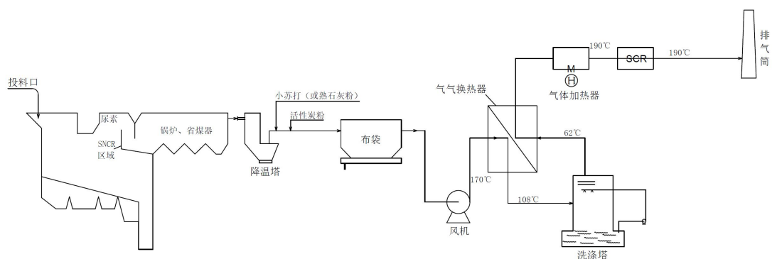
图 4 C 型生活垃圾焚烧烟气净化系统
