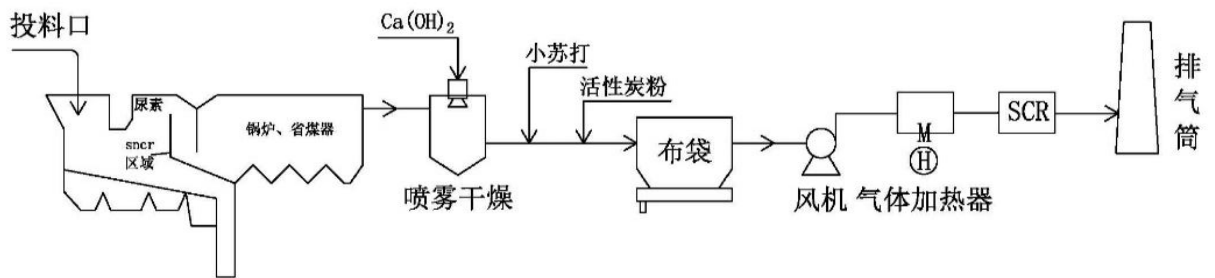
图6 E型生活垃圾焚烧烟气净化系统
