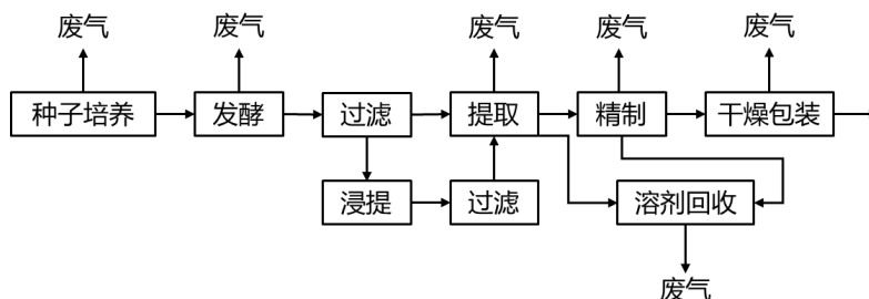
图 5.1 发酵类制药工艺流程及产污节点
