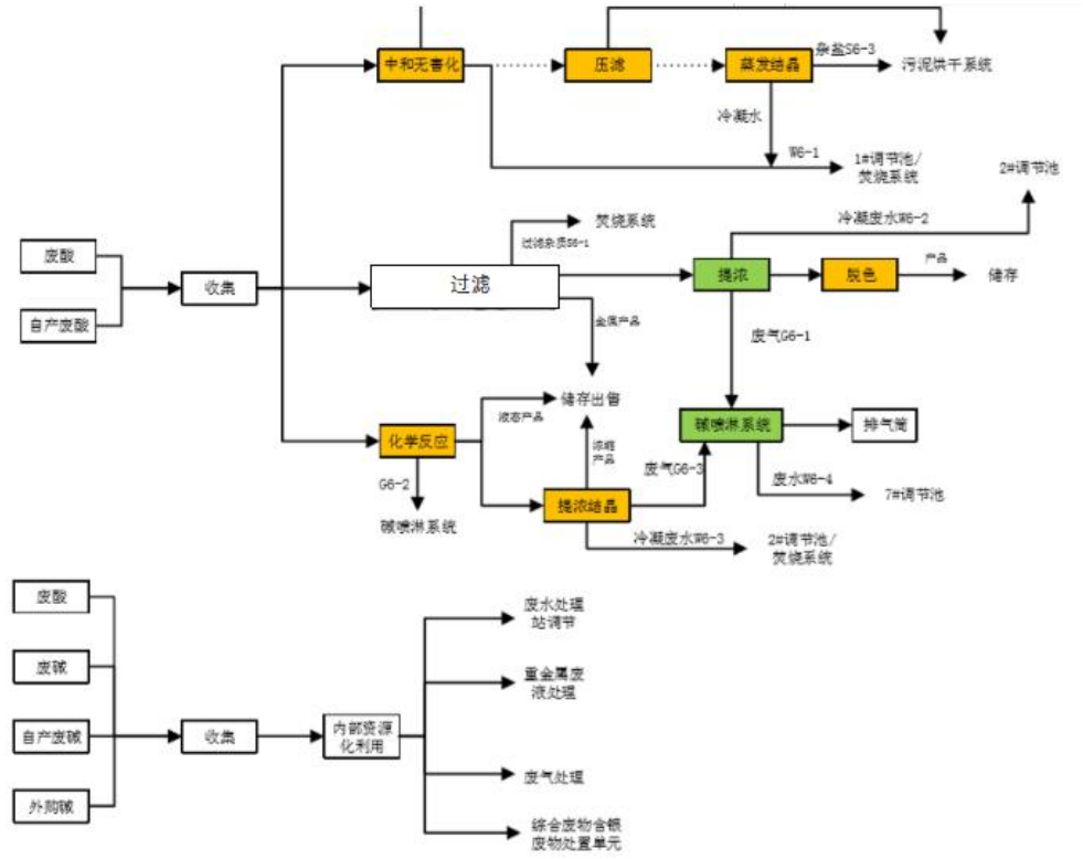
图 6 废酸、废碱处理工艺流程图
